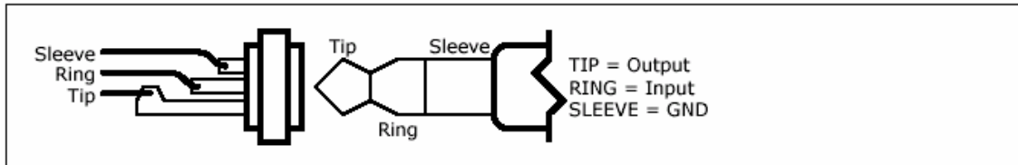
Esquema del cableado para la entrada TRS de ¼"
